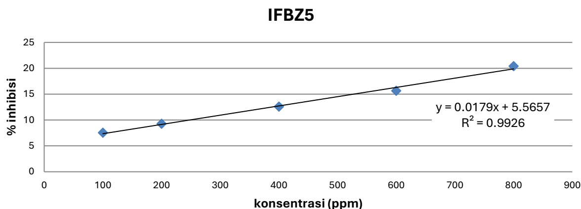
Gambar 2. Kurva Baku Serapan Isolat Fungi Endofit Kode IFBZ5 Pada Batang Tanaman Bidara ( Ziziphus mauritiana Lam.)
